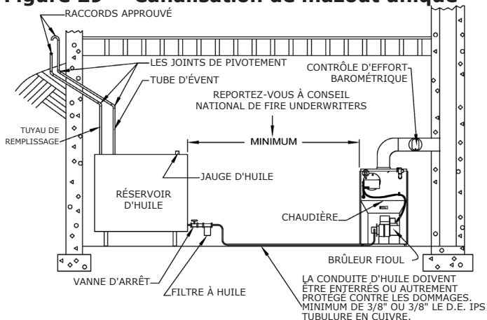
Figure 29 - Canalisation de mazout unique
