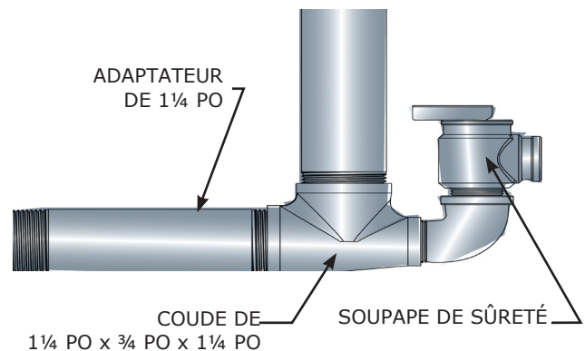
Figure 6 – Adaptateur raccordé au coude
