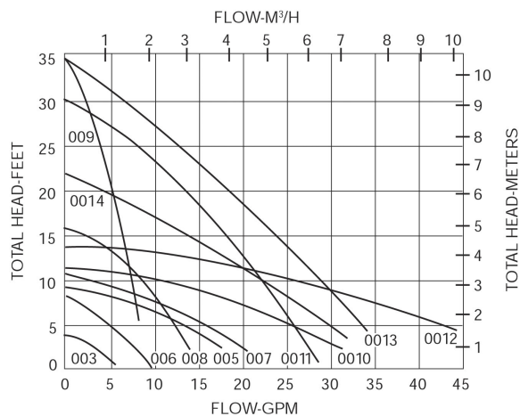
Figure 48 - Courbe de la pompe Taco
