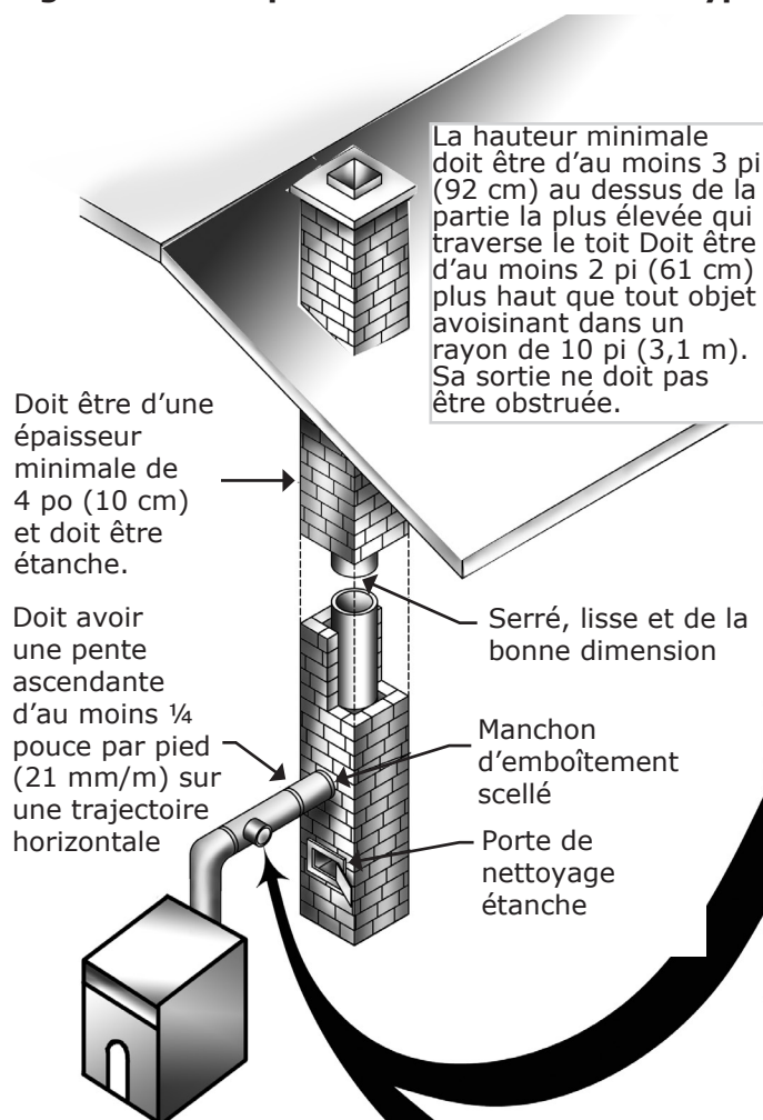
Figure 32 - Emplacements de cheminée types
