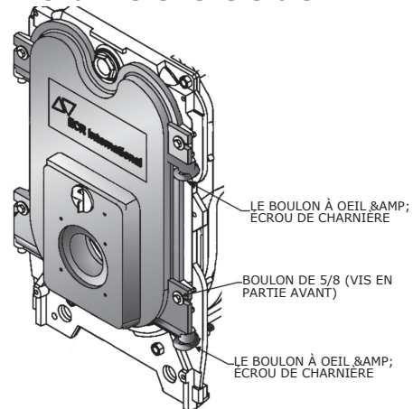
Figure 5 – Charnière réversible
