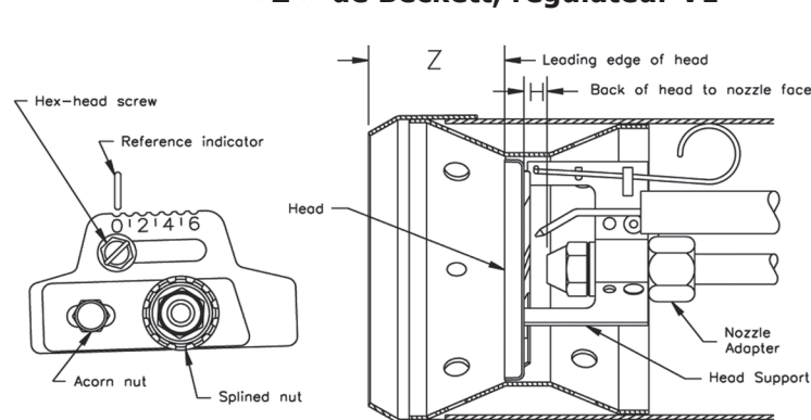
Figure 42 - Vérification/réglage de la dimension « Z » de Beckett, régulateur V1
