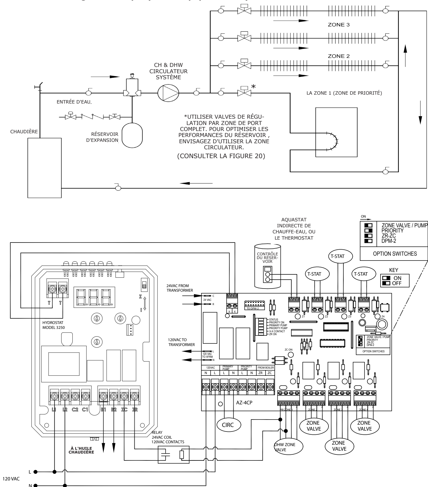
Figure 19 - Canalisations et câblage multizone avec soupapes de zones et priorité à l'eau chaude à usage domestique (avec soupape de zone)
