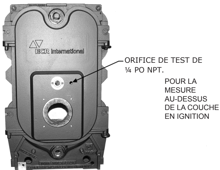
Figure 33 - Orifice à pression pour vérifier le tirage
