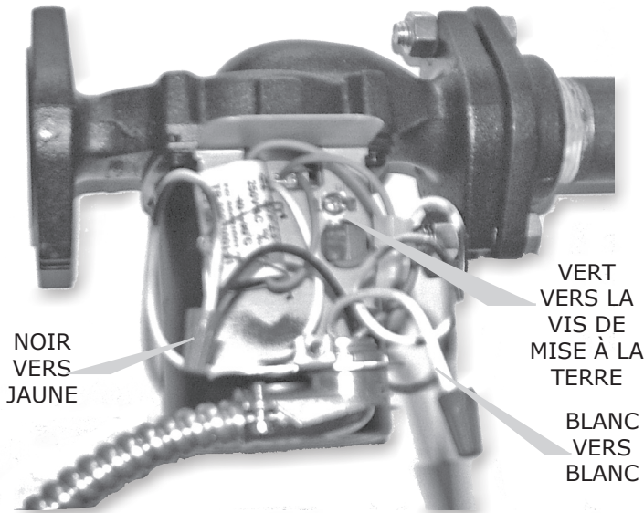
Figure 14 - Câblage du circulateur
