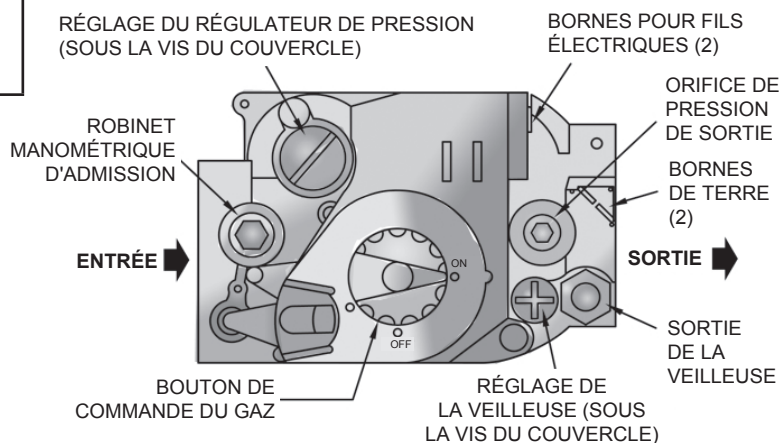
Figure 15 - Réglage de la flamme de la veilleuse
