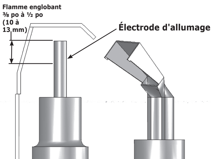
Figure 15 - Réglage de la flamme de la veilleuse
