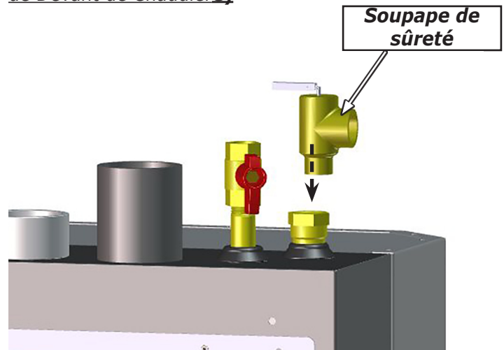
FIGURE 5-1 Soupape de sûreté et évant (A regardé de Devant de Chaudière)
