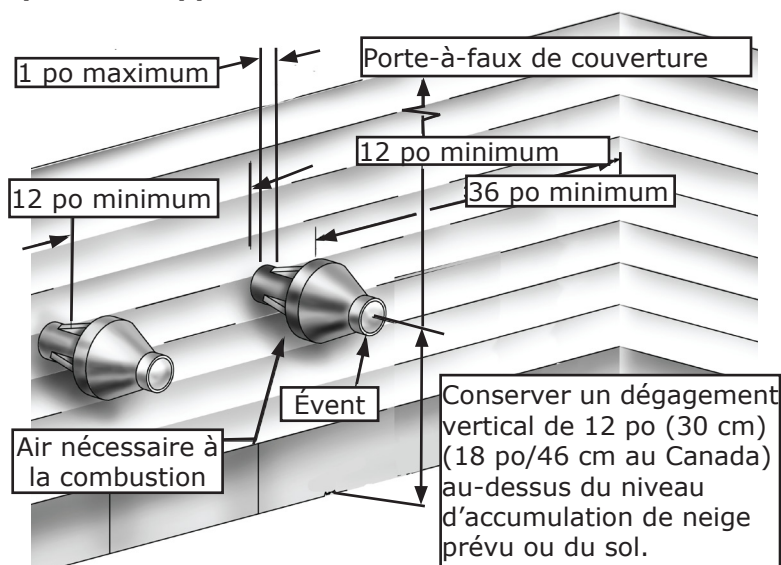
FIGURE 6-5 Paroi latérale Borne concentriques plusieurs appareils
