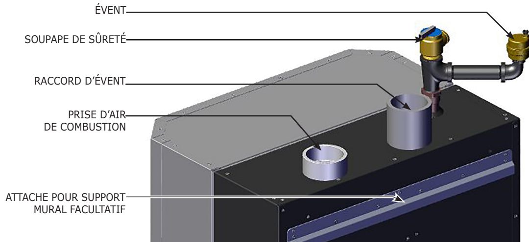
FIGURE 3-1 Composants de la chaudière
