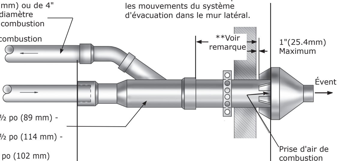
FIGURE 6-6 Extrémité d'évent concentrique
