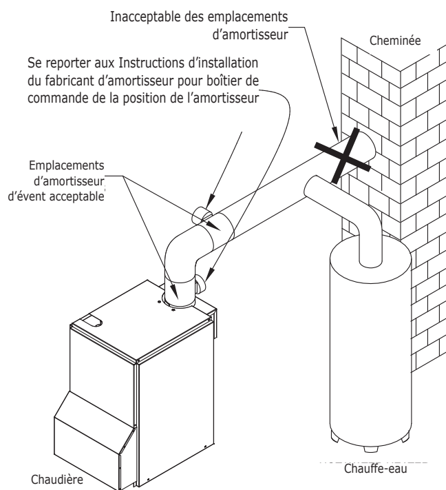
Figure 11 - Emplacement du registre d'évent
