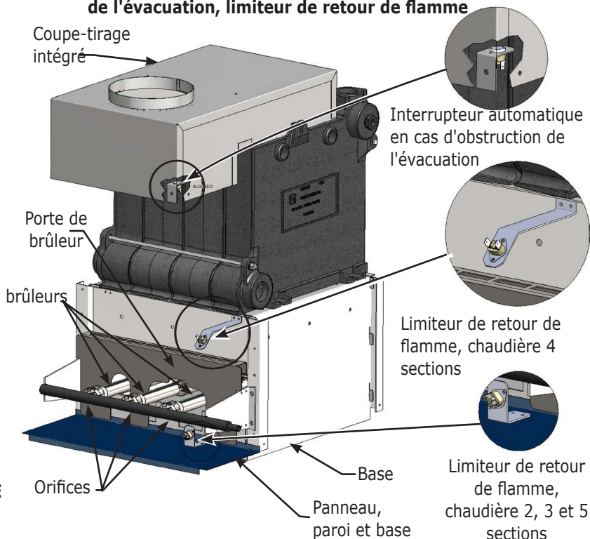
Figure 15 - Interrupteur manométrique en cas d'obstruction de l'évacuation, limiteur de retour de flamme
