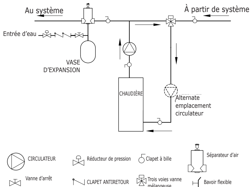
Figure 5 - Canalisation de dérivation : température fixe seulement avec soupape de zone
