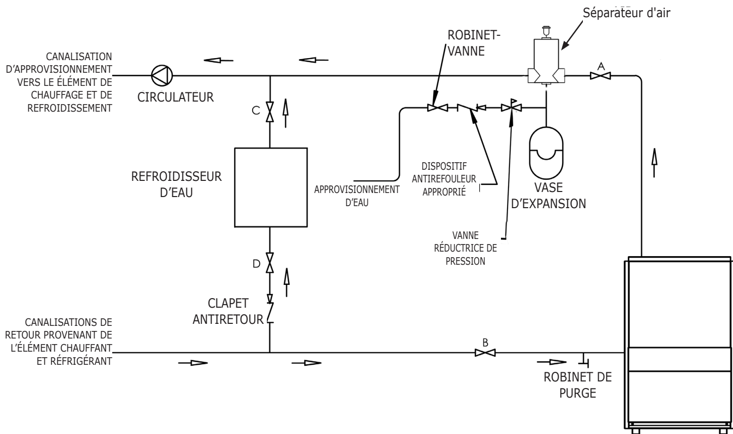
Figure 3 - Circulateurs fixés au système d'approvisionnement, chaudière utilisée dans une configuration avec système de réfrigération. Consulter les conditions spéciales en page 9.
