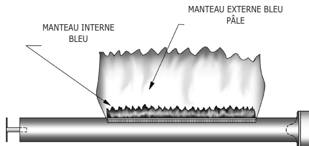
Figure 16 - Flamme du brûleur à gaz
