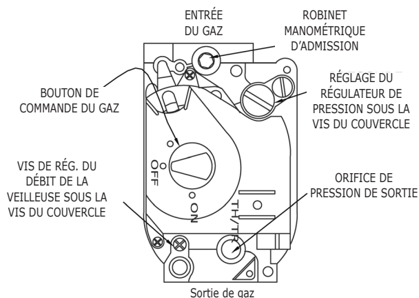
Figure 14 - Veilleuse intermittente
