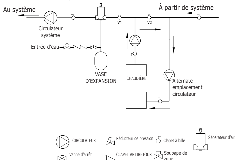
Figure 5 - Canalisation de dérivation : température fixe seulement avec soupape de zone
