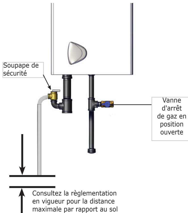
Figure 8 - Tuyauterie d'évacuation de la soupape de sécurité
