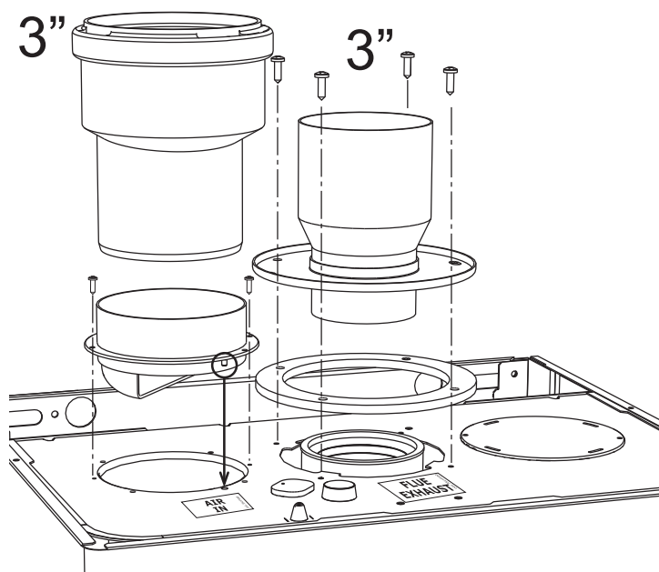
Figure 11 - Raccord d'air de combustion
