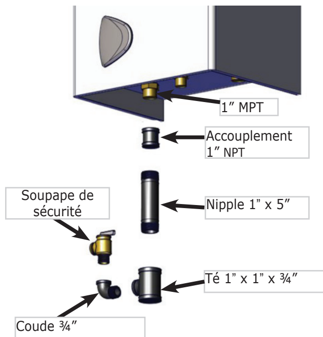
Figure 7 - Soupape de sécurité et évent d'air (vue de face à la chaudière)
