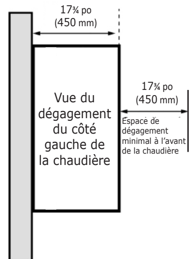
FIGURE 4-2c Dégagement pour l'entretien, installation dans un placard
