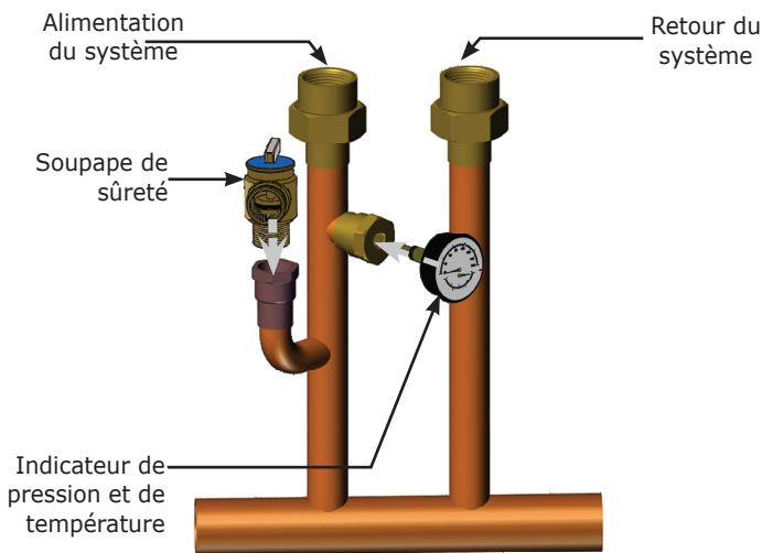
FIGURE 5-1 Soupape de sûreté
