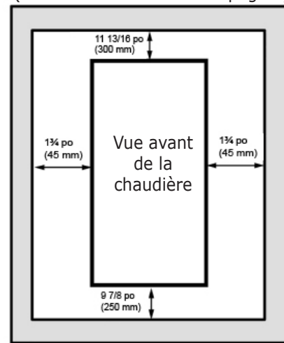
FIGURE 4-2b Dégagement pour l'entretien, côté gauche de la chaudière
