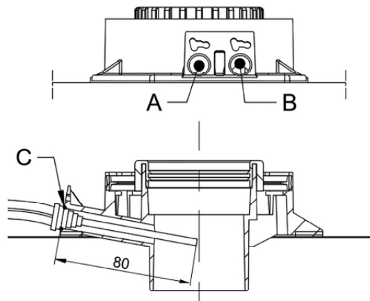
FIGURE 9-7 Orifice d'analyse de l'air nécessaire à la combustion et de la température
