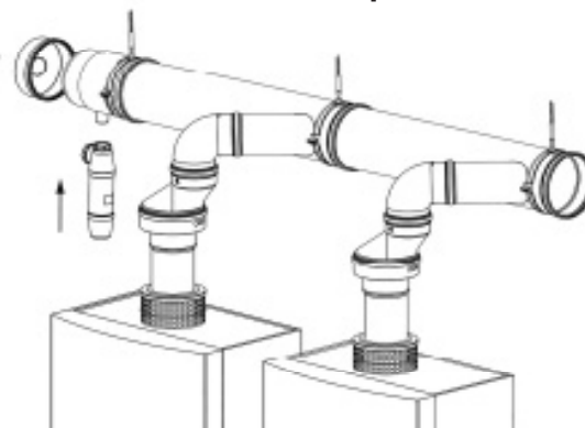
FIGURE 6-23 Installation adéquate des canalisations
