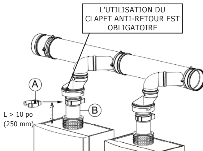
FIGURE 6-21 Installation adéquate des canalisations
