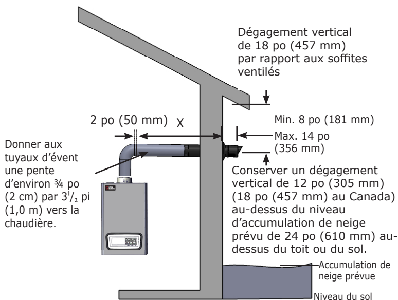
FIGURE 6-2 Événement coaxial pour mur latéral
