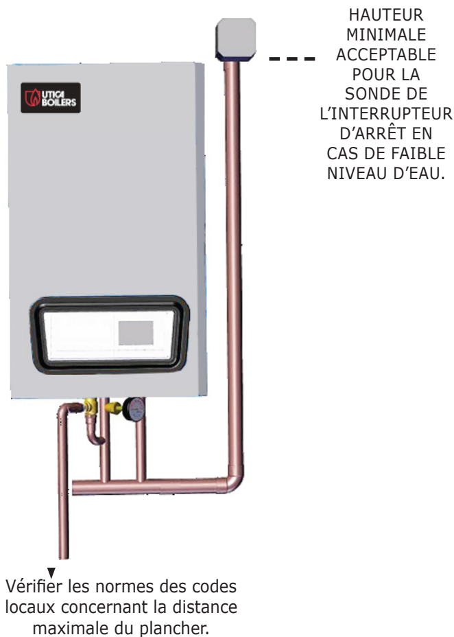
FIGURE 5-3 Canalisations du système : emplacement de la sonde de l'interrupteur en cas de faible niveau d'eau
