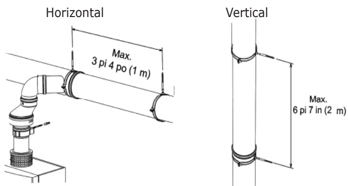
FIGURE 6-25 Distance maximale entre les supports
