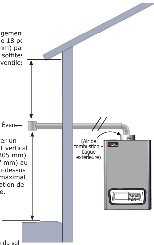
FIGURE 6-14 Évacuation murale, prise intérieure d'air nécessaire à la combustion
