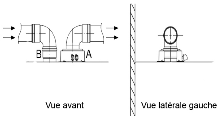
FIGURE 6-6 Options d'installation d'extrémités d'évent horizontales séparées
