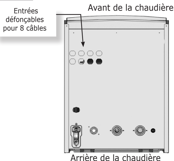
FIGURE 8-1 Entrées défonçables au bas de la chaudière
