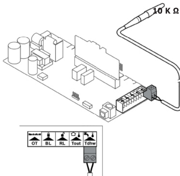
FIGURE 8-12 Thermostat indirect 10 k \Omega pour chauffe-eau
