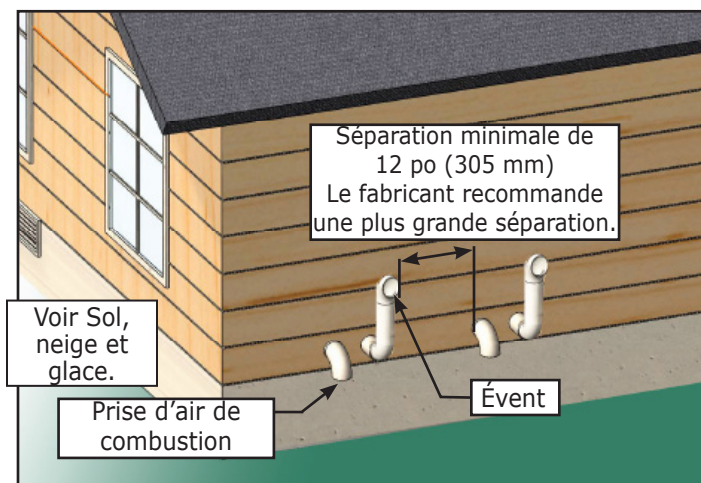
FIGURE 6-9 Évent latéral double (plusieurs appareils)
