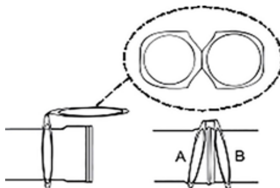
FIGURE 6-4 – Raccordement à attache mécanique pour conduite de carburant double
