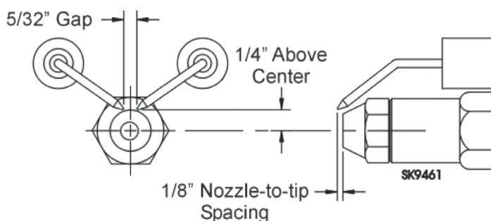
Figure 40 - Réglages de la pointe d'électrode Beckett AFG pour chaudières à trois passages
