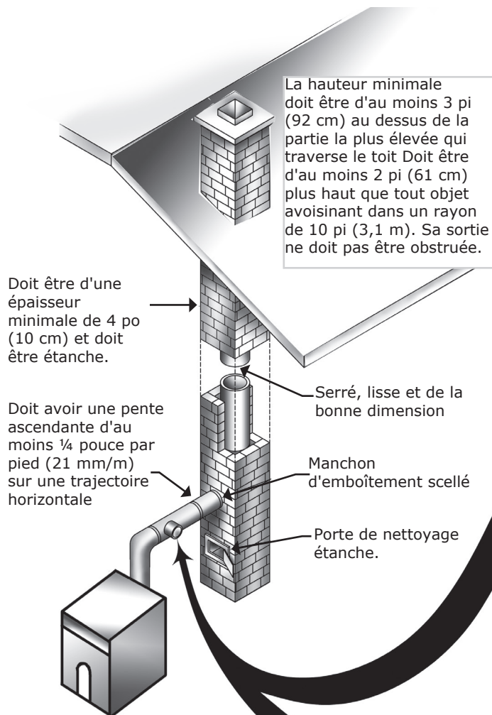
Figure 32 - Emplacements de cheminée types
