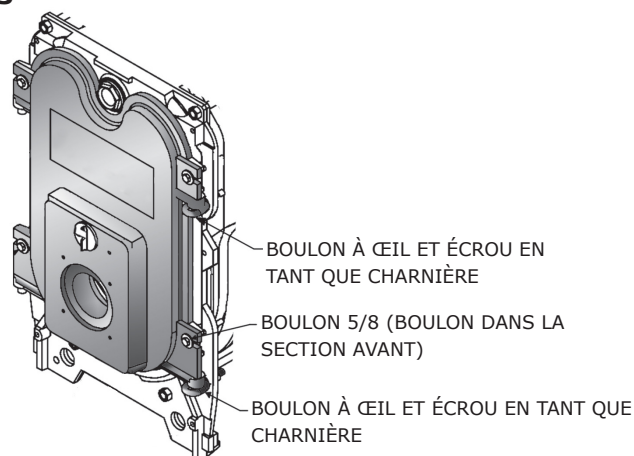
Figure 5 – Charnière réversible
