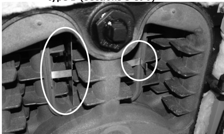
Figure 13a - Déflecteurs de troisième passage de type B (sections 5 et 6)
