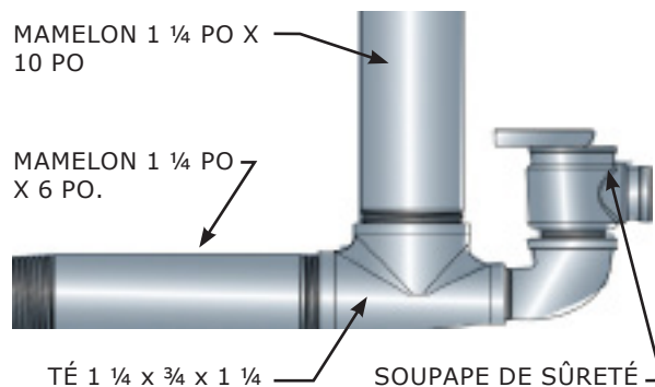
Figure 6 - Canalisation d'approvisionnement
