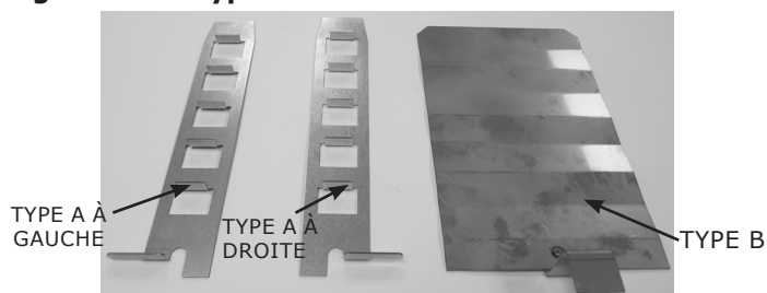
Figure 13c - Types de déflecteurs A et B
