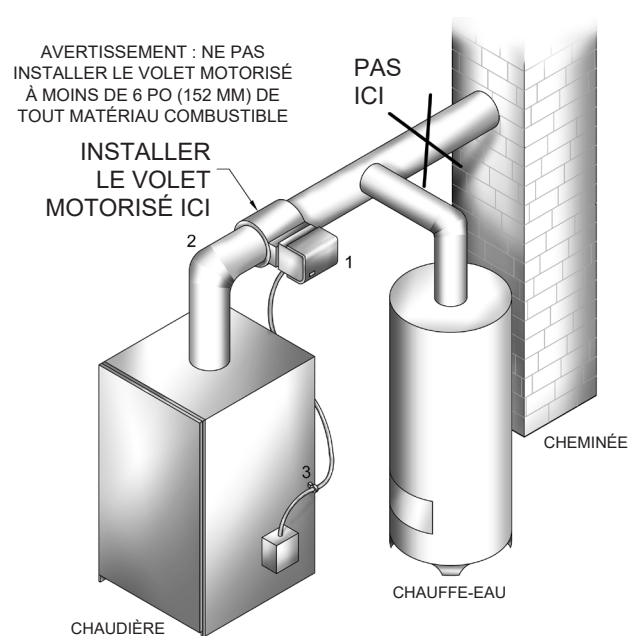
Figure 9 - Emplacement du volet motorisé
