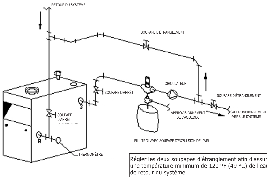
Figure 7 - CANALISATION DE DÉRIVATION; CIRCULATEUR AU RETOUR
