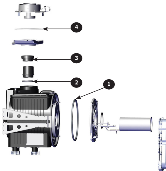
KIT 550003156 - KITS DE REMPLACEMENT DU JOINT DE LA CHAMBRE DE COMBUSTION 125/150 - KIT COMPREND:
