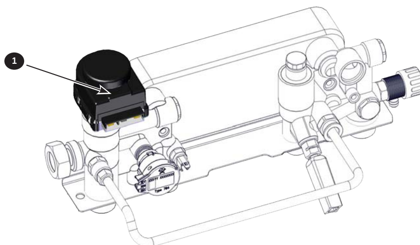
KIT 550003166 - MOTEUR DE VANNE 3 VOIES - KIT DE REMPLACEMENT - 125/150 KIT COMPREND:
