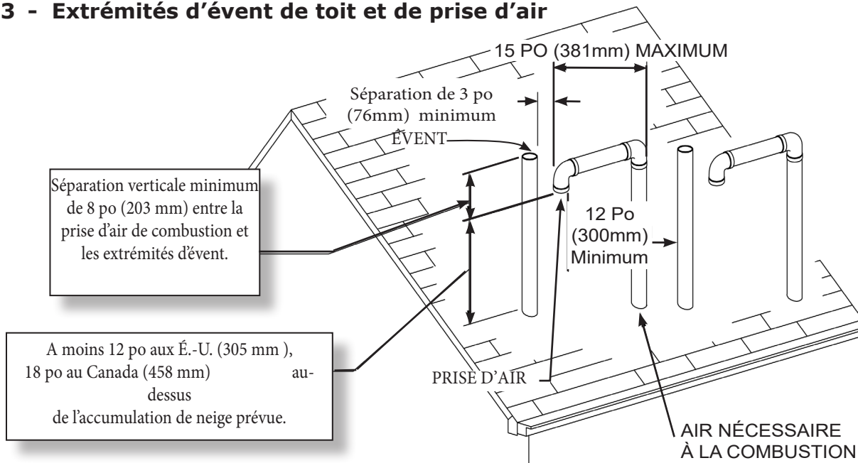
Figure 13 - Extrémités d'évent de toit et de prise d'air
