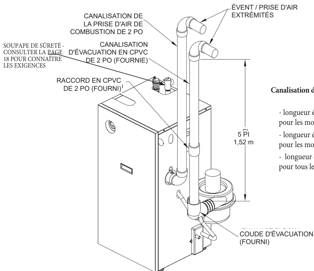
Figure 19 - Prise d'air de combustion et évent - Raccordements à la chaudière
