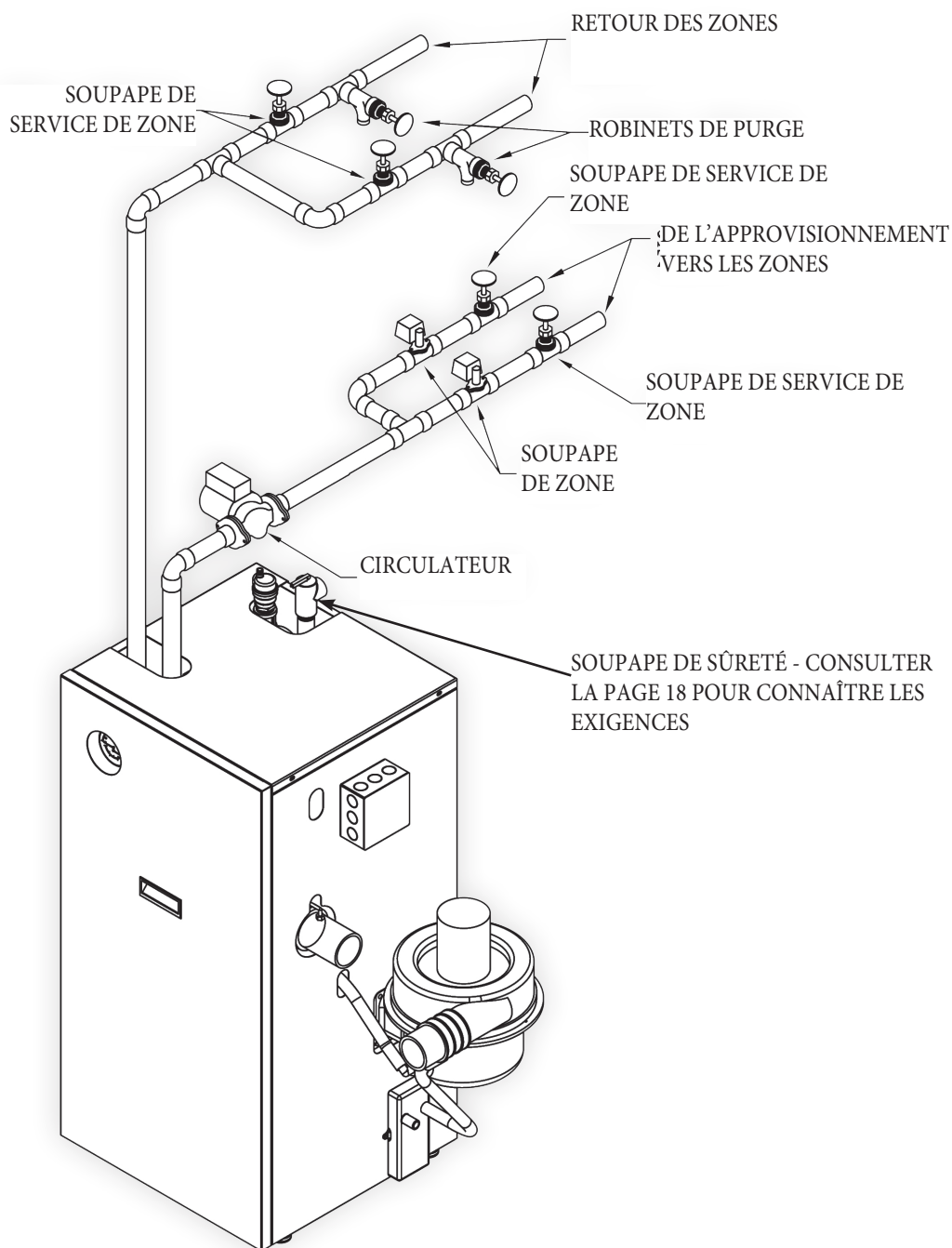
Figure 4 - Canalisations à deux zones de la chaudière avec soupapes de zone
