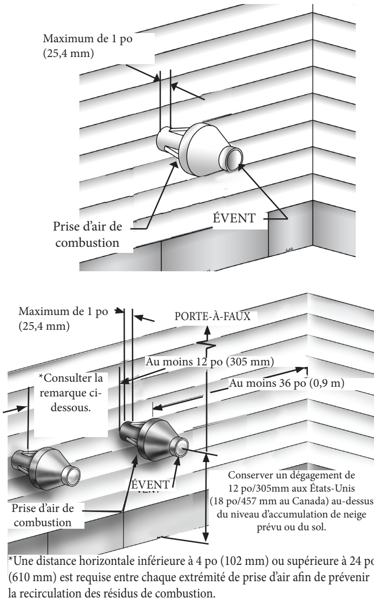
Figure 18 - Extrémités d'évent concentrique
