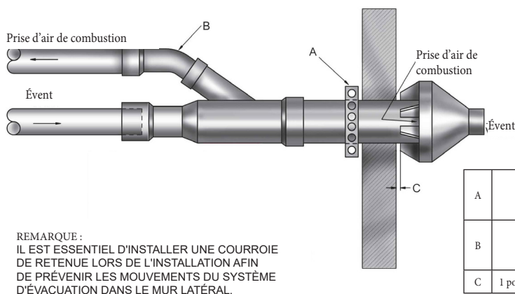
Figure 16 - Extrémités d'évent concentrique
