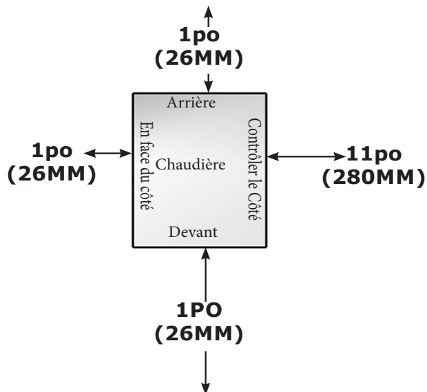
Figure 2 -Les Dégagements minimums A la Construction Combustible
