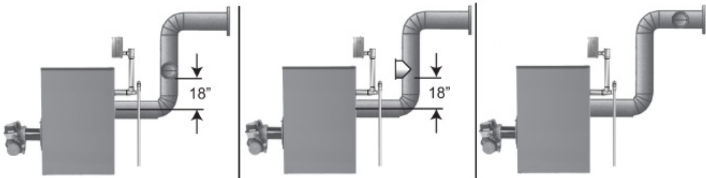
Figure 31 - Emplacements adéquats du régulateur de tirage
