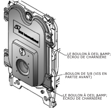
Figure 5 – Charnière réversible
