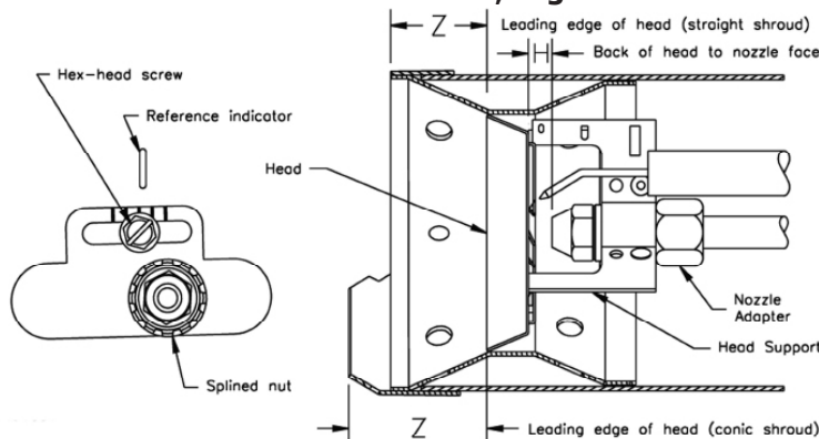
Figure 41 - Vérification/réglage de la dimension « Z » de Beckett, régulateurs L1 et L2
