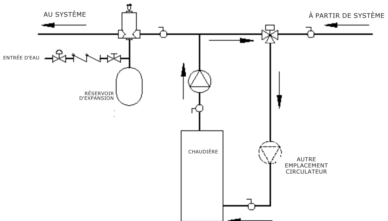
Figure 25 - Canalisation de dérivation (soupape de mélange automatique)
