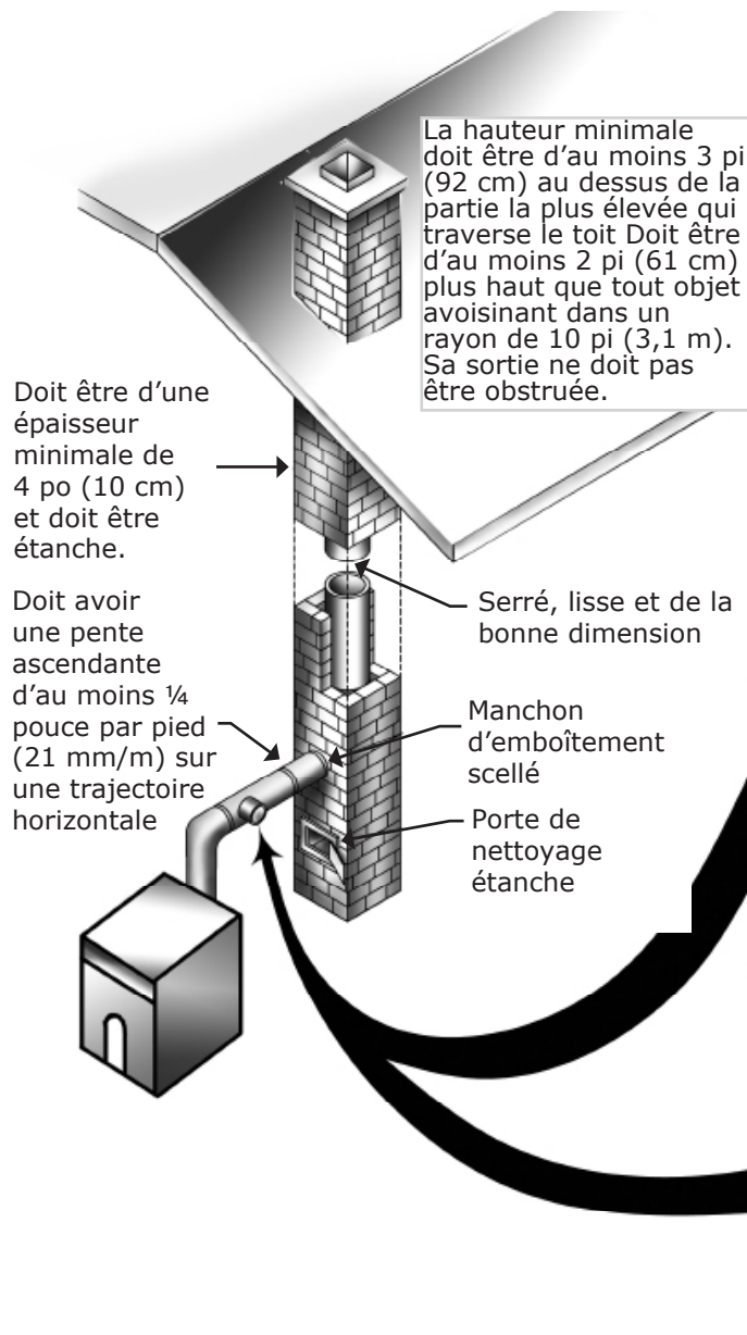
Figure 32 - Emplacements de cheminée types
