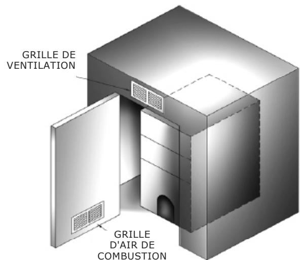
Figure 3 – Prises d’air pour une chaudière située dans un espace restreint (pièce d’entretien)
