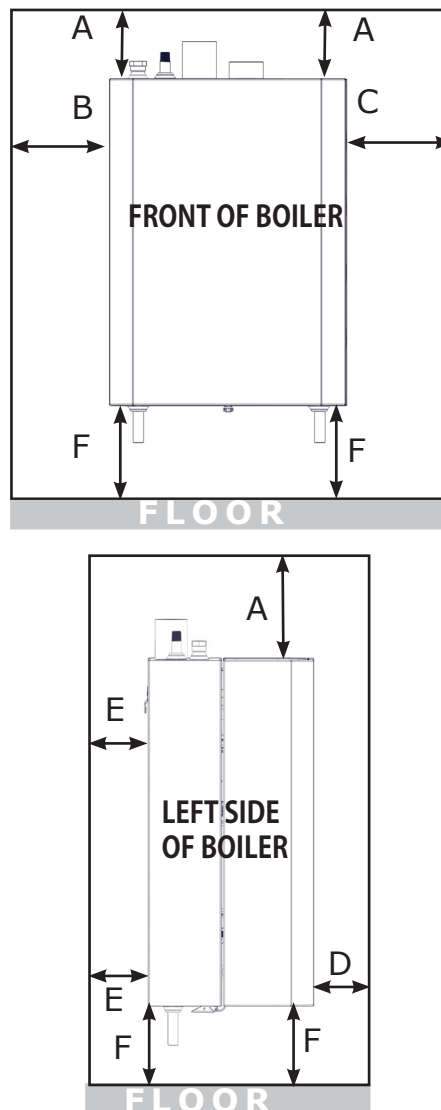
FIGURE 4-1 Dégagement par rapport aux matériaux combustibles
