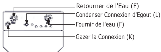
Vue inférieure Identification liaison 150-299 MBH
