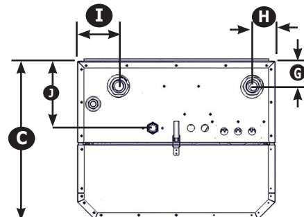
Vue de dessous dimensions 299 MBH
