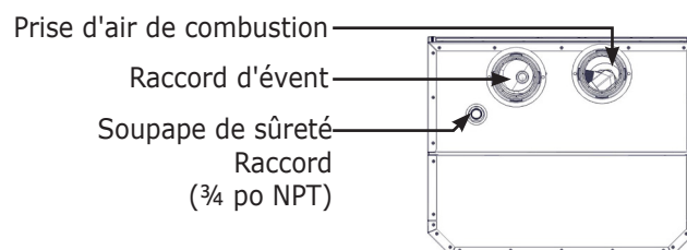
Vue inférieure Identification liaison 150-299 MBH
