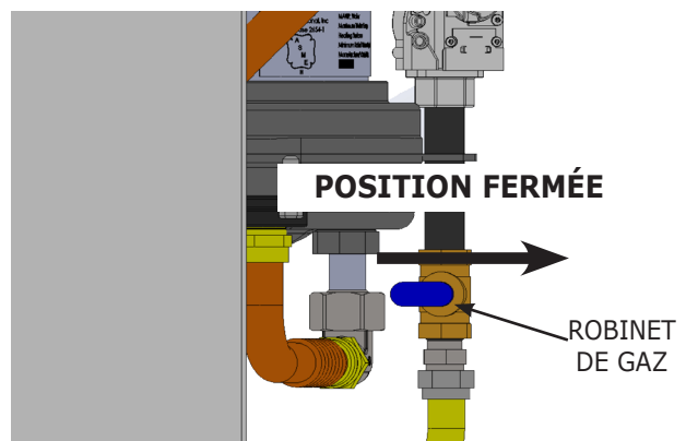
FIGURE 10-2 Robinet de gaz - modèle 299 MBH
