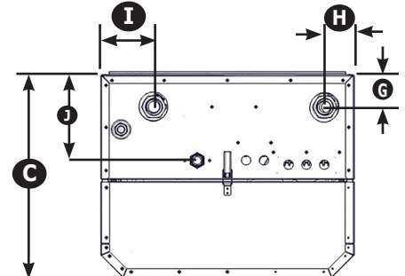
Vue de dessous dimensions 299 MBH
