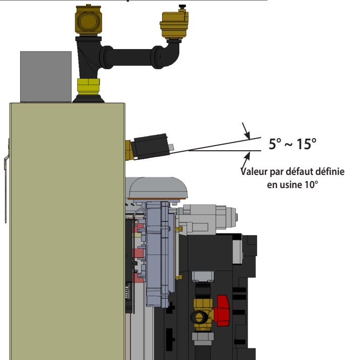
FIGURE 4-3 faible coupure eau Orientation
