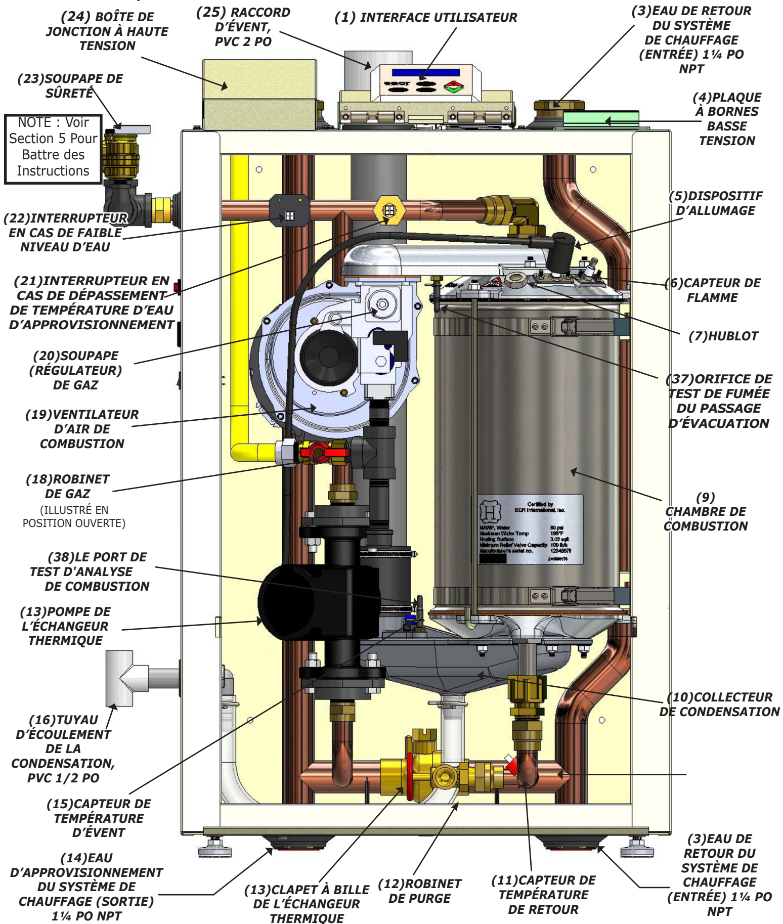
FIGURE 3-2 Composants de la chaudière
