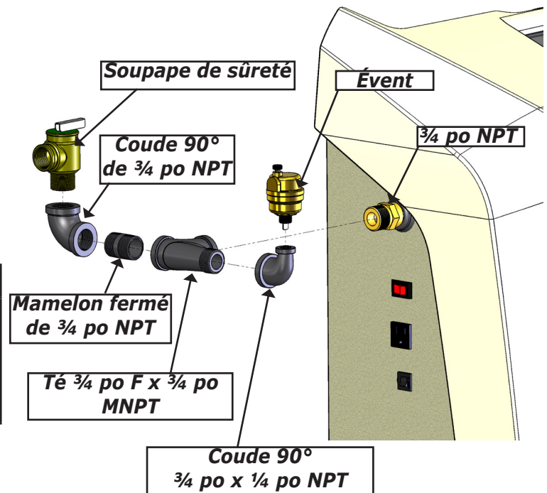
FIGURE 5-1 Soupape de sûreté et évent
