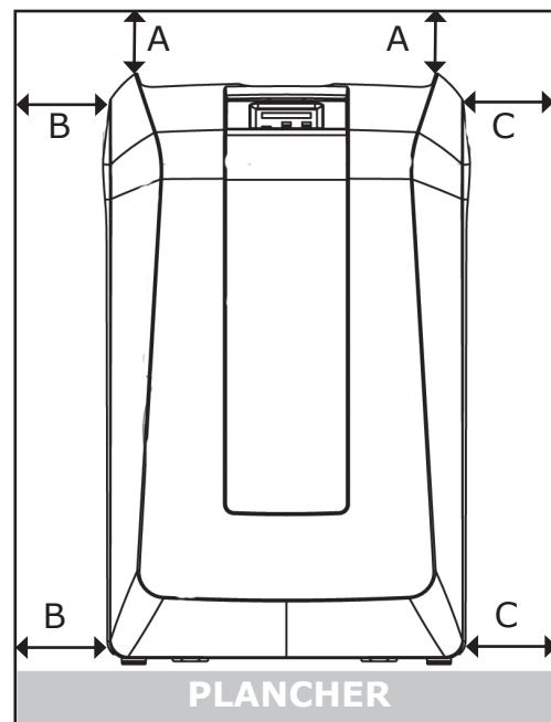
FIGURE 4-1 Dégagement par rapport aux matériaux combustibles
