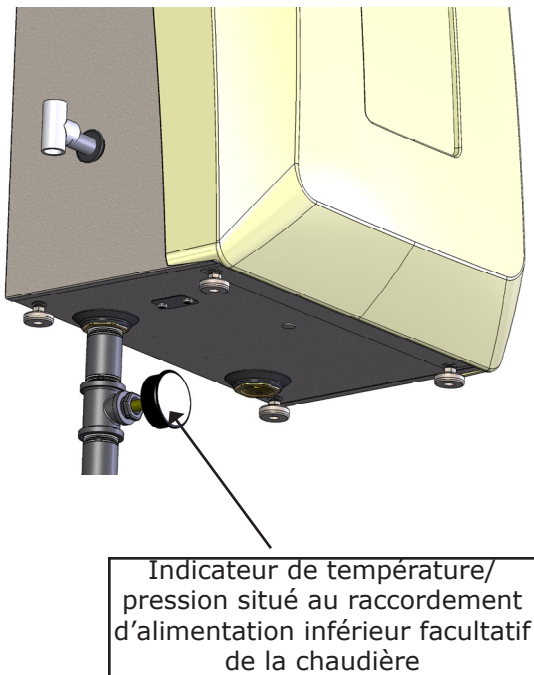
FIGURE 5-3 Installation de l'indicateur de température/pression
