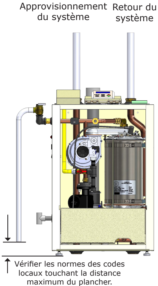
FIGURE 5-4 Canalisations du système
