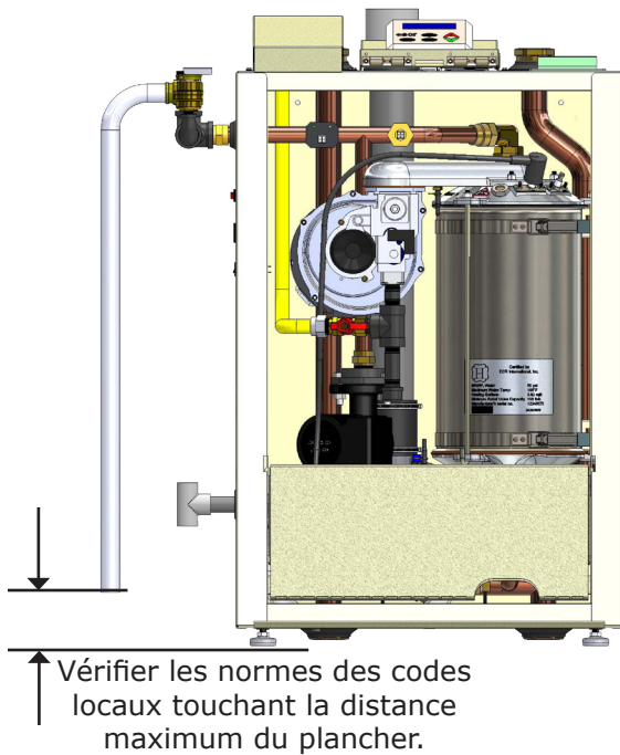
FIGURE 5-3 Installation de l'indicateur de température/pression
